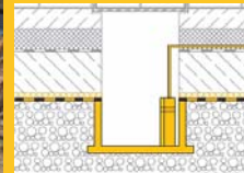
Смотровая шахта с насосом для откачивания воды:
